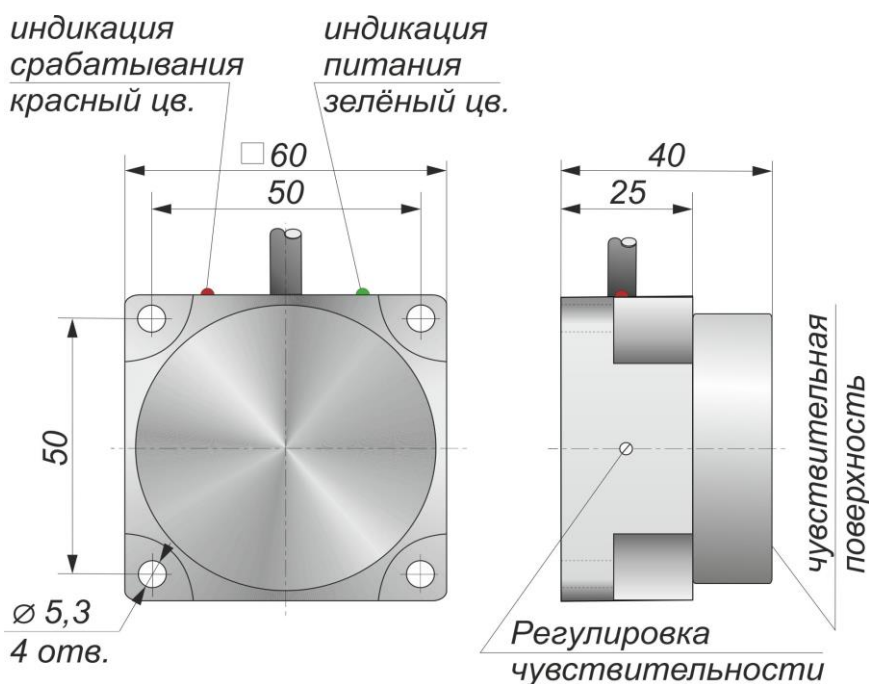
Габаритный чертеж
